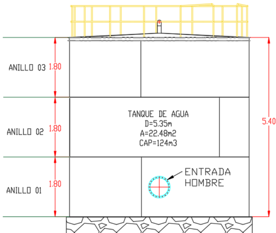
FIG. N°3: Composición del tanque por Anillos.
