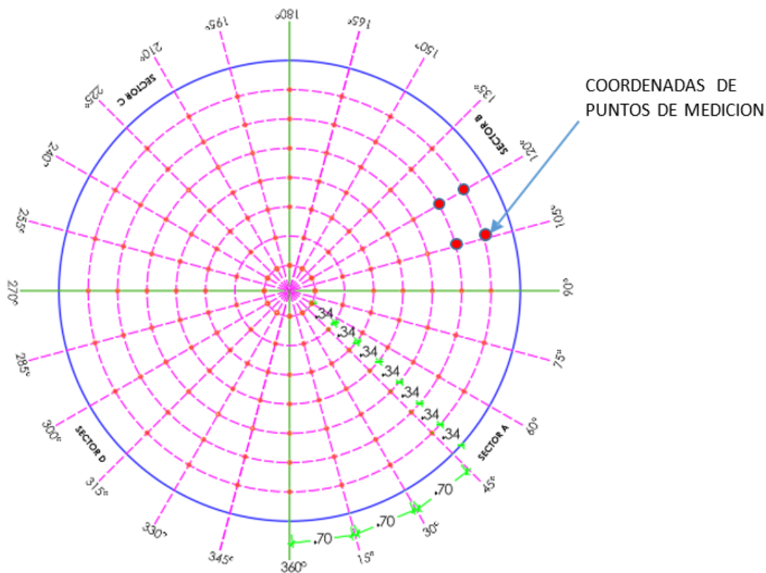
FIG. N°5: Distribución de puntos de medición en fondo de Tanque.
