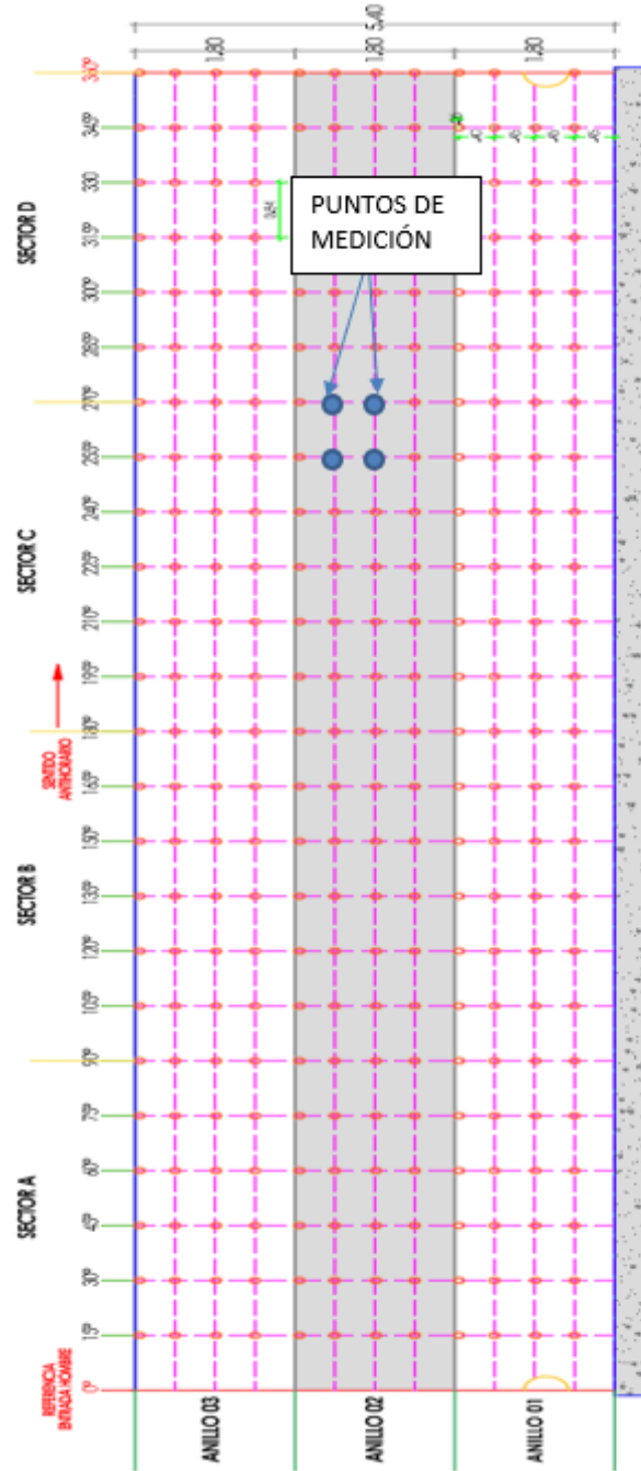
FIG. N°4: Distribución de puntos de medición en manto lateral del tanque - 240 puntos.
