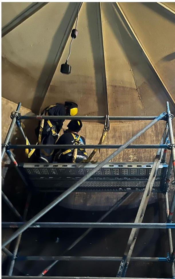
FIG. N°6: Aplicación de grasa y silicona en cada uno de los puntos a medir. (Evidencia fotográfica de medición de puntos en el manto lateral).
